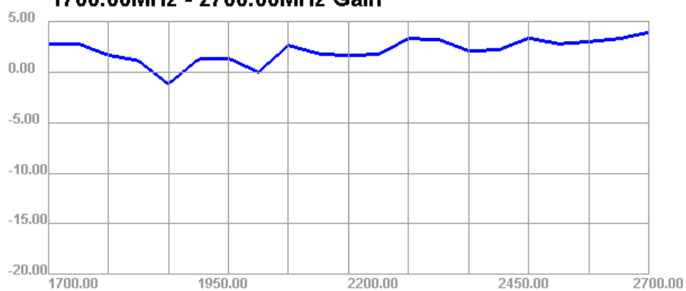
1700.00MHz - 2700.00MHz Gain
