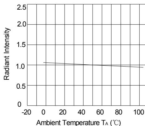
Fig.4 环境温度VS.相对亮度
