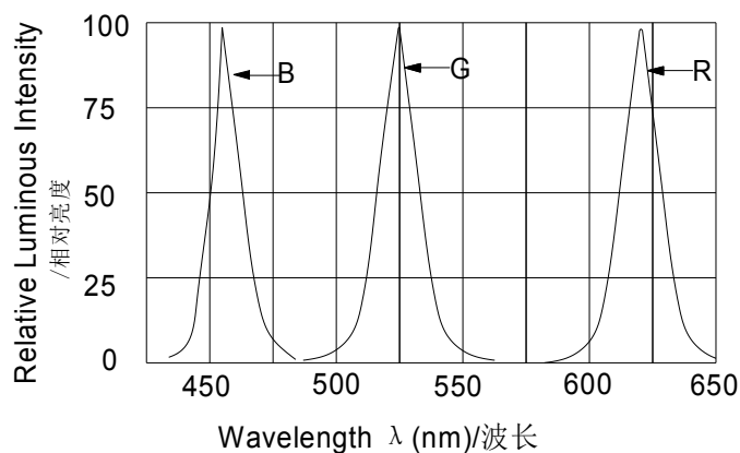
Fig.5 相对亮度 Vs. 波长
