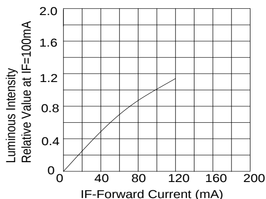
Fig.2 相对亮度 Vs. 正向电流
