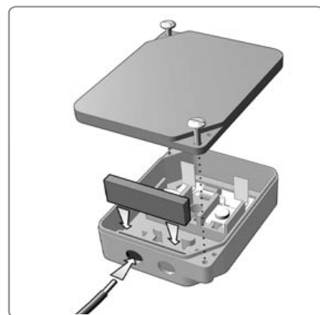
Cableado de caja de conexión ProCharger™ S
