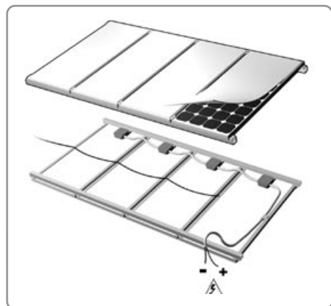
Cubra el módulo con material opaco durante la instalación
