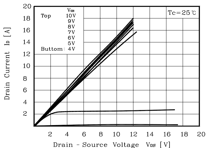
Fig. 1 I_D - V_{DS}
