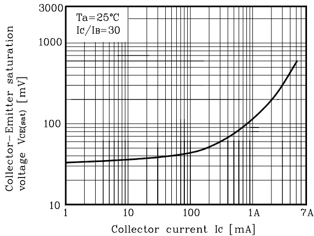
Fig. 3 V_{CE(sat)} - I_C
