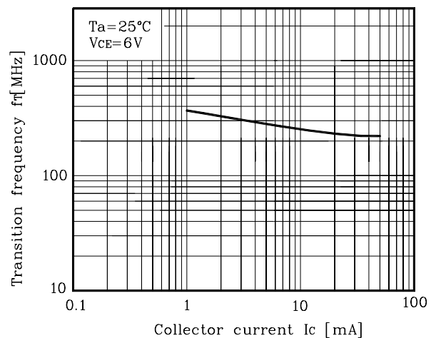
Fig. 4 f_T - I_C
