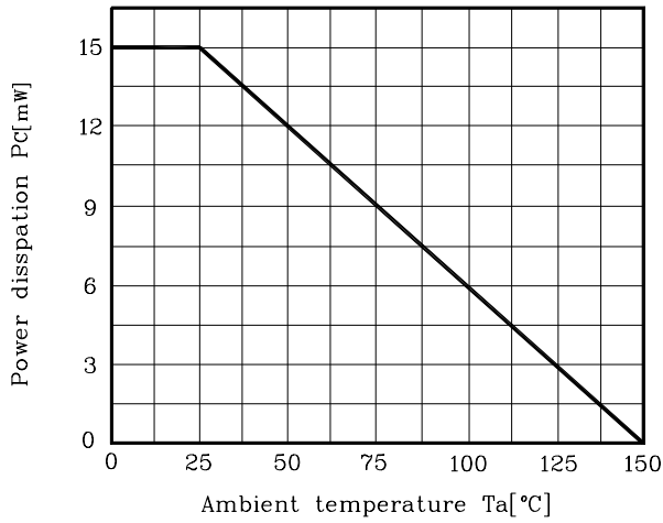
Fig. 1 P_c - T_a
