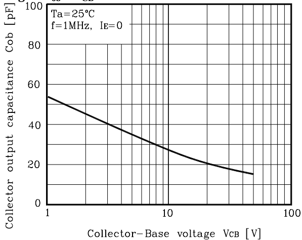
Fig. 5 C_{ob} - V_{CB}
