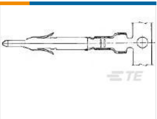
TE Model / Part #170363-1 MINI UNIVERSAL M-N-L PIN LP
