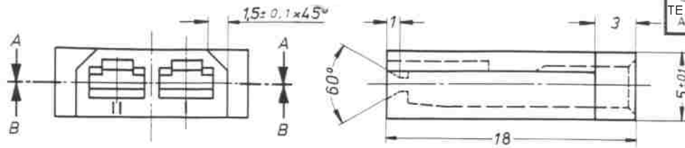
Schnitt B-B
